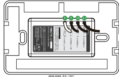
開關背面
